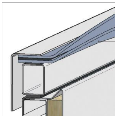
Rys. 39 Wypełnienie kłapy: 2-warstwowa kopia akrylowa
