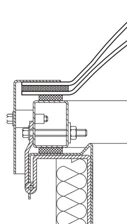
Rys. 40 Przekrój przez kłapę, wypełnienie: 2-warstwowa kopia akrylowa
