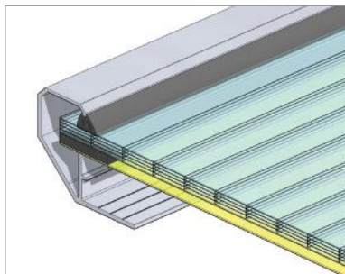
Rys. 131 Wypełnienie pasma: płyta z poliwęglanu komorowego (PCA 10), płyta NRO, przedzielone pustką powietrzną (PP)
