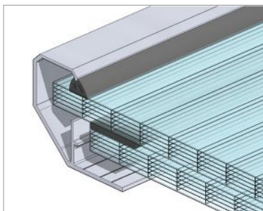
Rys. 127 Wypełnienie pasma: dwie płyty z poliwęglanu komorowego (PCA 16 + PCA 16) przedzielone pustką powietrzną (PP)
