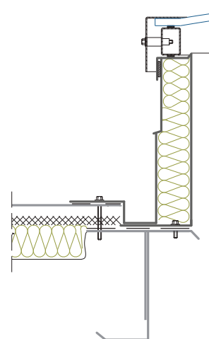
Rys. 80 Montaż klapy z podstawą PR, przekrój równoległy do spadku dachu od strony okapu
