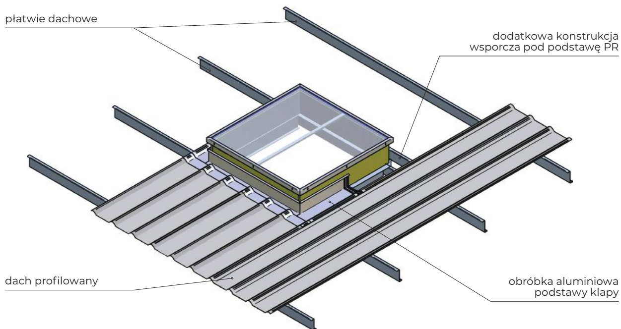
Rys. 77 Montaż klapy oddymiającej z podstawą PR na dachu profilowanym
