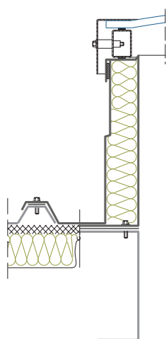
Rys. 78 Montaż klapy z podstawą PR, przekrój prostopadły do spadku dachu
