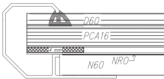
Rys. 135 Przekrój przez pasmo o szerokości 1,5÷4,0 m; rama nośna (N) i rama dociskowa (D) o szerokości 60 mm
