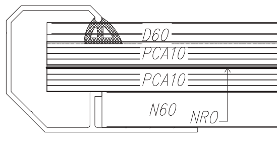
Rys. 139 Przekrój przez pasmo o szerokości 1,2÷3,5 m; rama nośna (N) i rama dociskowa (D) o szerokości 60 mm
