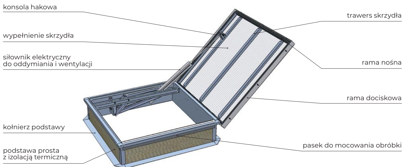
Rys. 57 Budowa klapy oddymiającej mcr PROLIGHT z przesuniętym sterowaniem elektrycznym do oddymiania i wentylacji, z opcją wyjścia na dach
