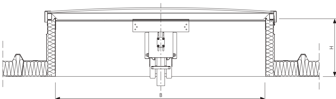
Rys. 75 Przekrój poprzeczny przez klapę mcr PROLIGHT typ E z podstawą PR do dachów profilowanych, prostopadłe do spadku dachu
