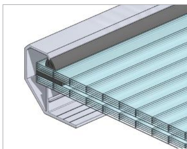
Rys. 122 Wypełnienie pasma: dwie płyty z poliwęglanu komorowego (PCA10 + PCA10) przedzielone pustką powietrzną (PP)
