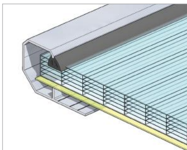
Rys. 129 Wypełnienie pasma: płyta z poliwęglanu komorowego (PCA), płyta NRO
