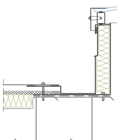
Rys. 79 Montaż klapy z podstawą PR, przekrój równoległy do spadku dachu od strony kalenicy
