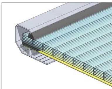
Rys. 134 Wypełnienie pasma: płyta z poliwęglanu komorowego (PCA 16), płyta NRO, przedzielone pustką powietrzną (PP)
