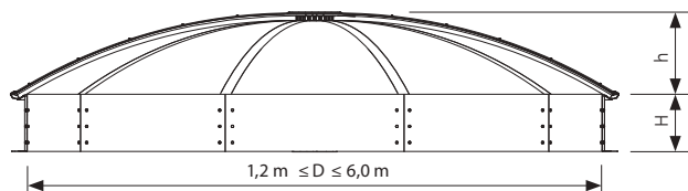
Rys. 111 Przekrój poprzeczny A-A przez świetlik kopułowy mcr PROLIGHT
