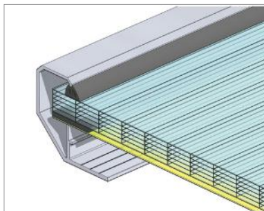
Rys. 136 Wypełnienie pasma: płyta z poliwęglanu komorowego (PCA 20), płyta NRO, przedzielone pustką powietrzną (PP)
